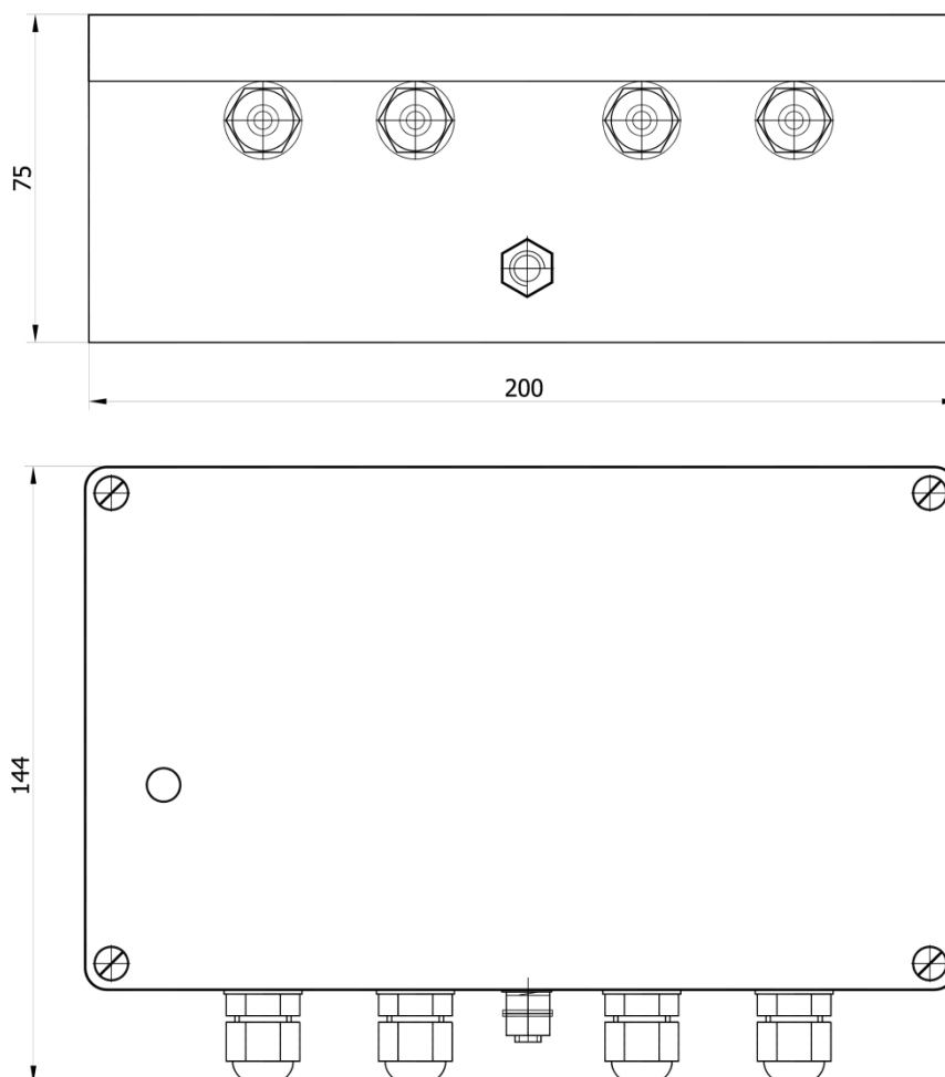
Рисунок 1 - Габаритный чертеж корпуса
